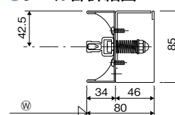
●レール部詳細図
