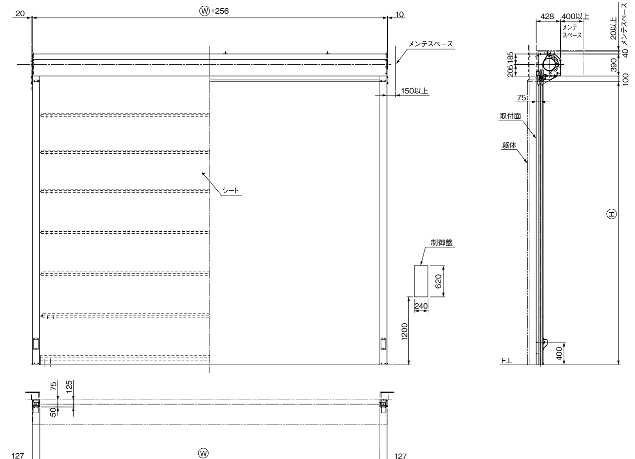
参考納まり図 単位:mm
