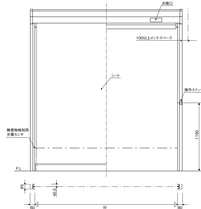
参考納まり図 単位:mm
