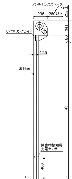
●レール部詳細図
